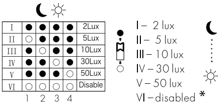
Fig. 3a: SMC-SEN
