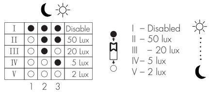
Fig. 3b: SMCB-SEN
