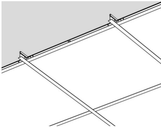
Sichtbare Tragschienen
