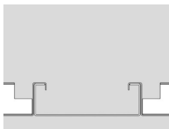
Armstrong gehängt
