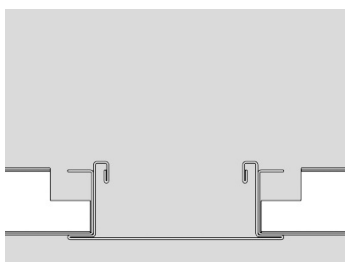
Armstrong gelegt
